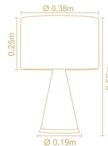
ABAJUR CONE Ref. 3195 Altura 0,56m Cúpula 0,25x0,38m Porta Lâmpada E27
