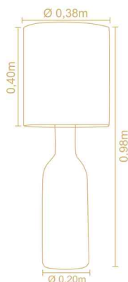
ABAJUR BOTTLE Ref. 3190 Altura 0,98m Cúpula 0,40x0,38m Porta Lâmpada E27
