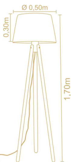
LUMINÁRIA DE PISO TRIPPÉ Ref. 2963/... Altura 1,70m Cúpula 0,30x0,50m Porta Lâmpada E27
