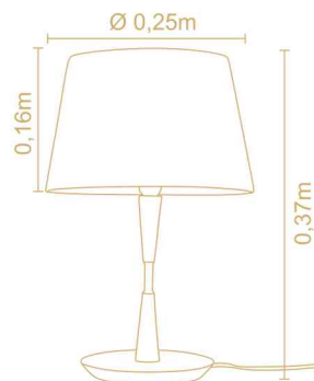
ABAJUR STANDARD PEQUENO Ref. 3025/... Altura 0,37m Cúpula 0,16x0,25m Porta Lâmpada E27
