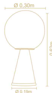
ABAJUR ESPHERA Ref. 3189 Altura 0,62m Porta Lâmpada E27
