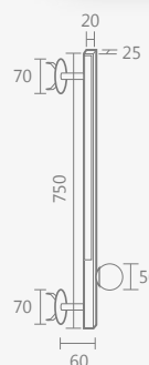
1017/2 – perfil print arandela LED mini globo
