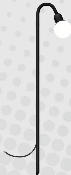
BALIZADOR SPHERA GLOBE 1349 Porta lâmpada: 1 x G9 Halopin Difusor: Globo de vidro branco opalino Ø 100 mm Luminária total: Ø 200 x \Phi 800 mm
