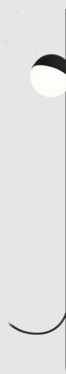
BALIZADOR SPHERA HALF 1344 Porta lâmpada: 1 x G9 Halopin Difusor: Globo de vidro branco opalino Ø 100 mm Luminária total: Ø 110 x \Phi 800 mm
