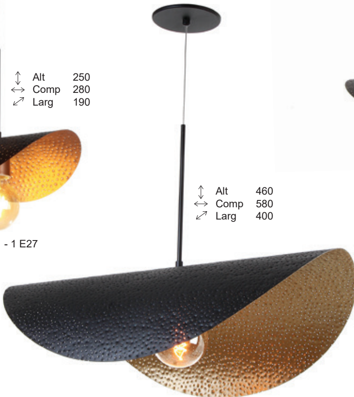
PD 5719 - 1 E27
