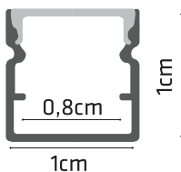
DESENHO TÉCNICO
